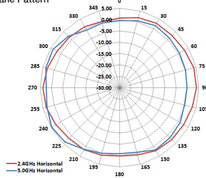
H-Plane Pattern
