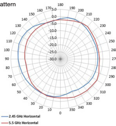
H-Plane Pattern
