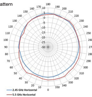
H-Plane Pattern
